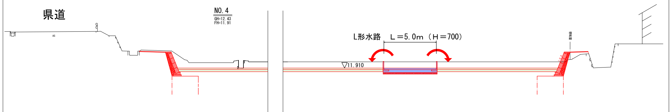
標準横断図 (NO. 4)
