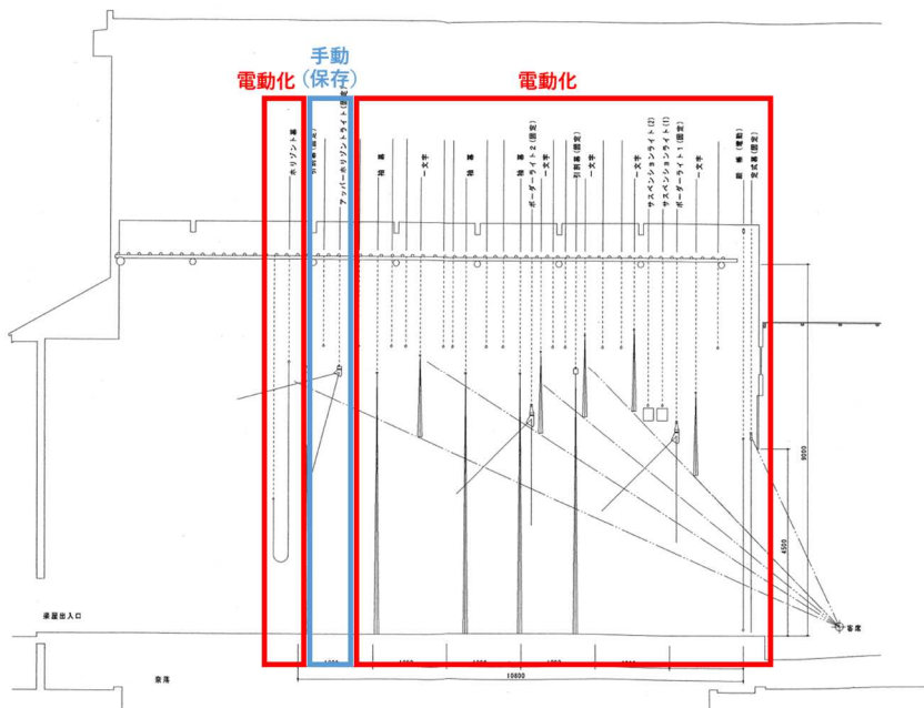
【舞台断面図】
