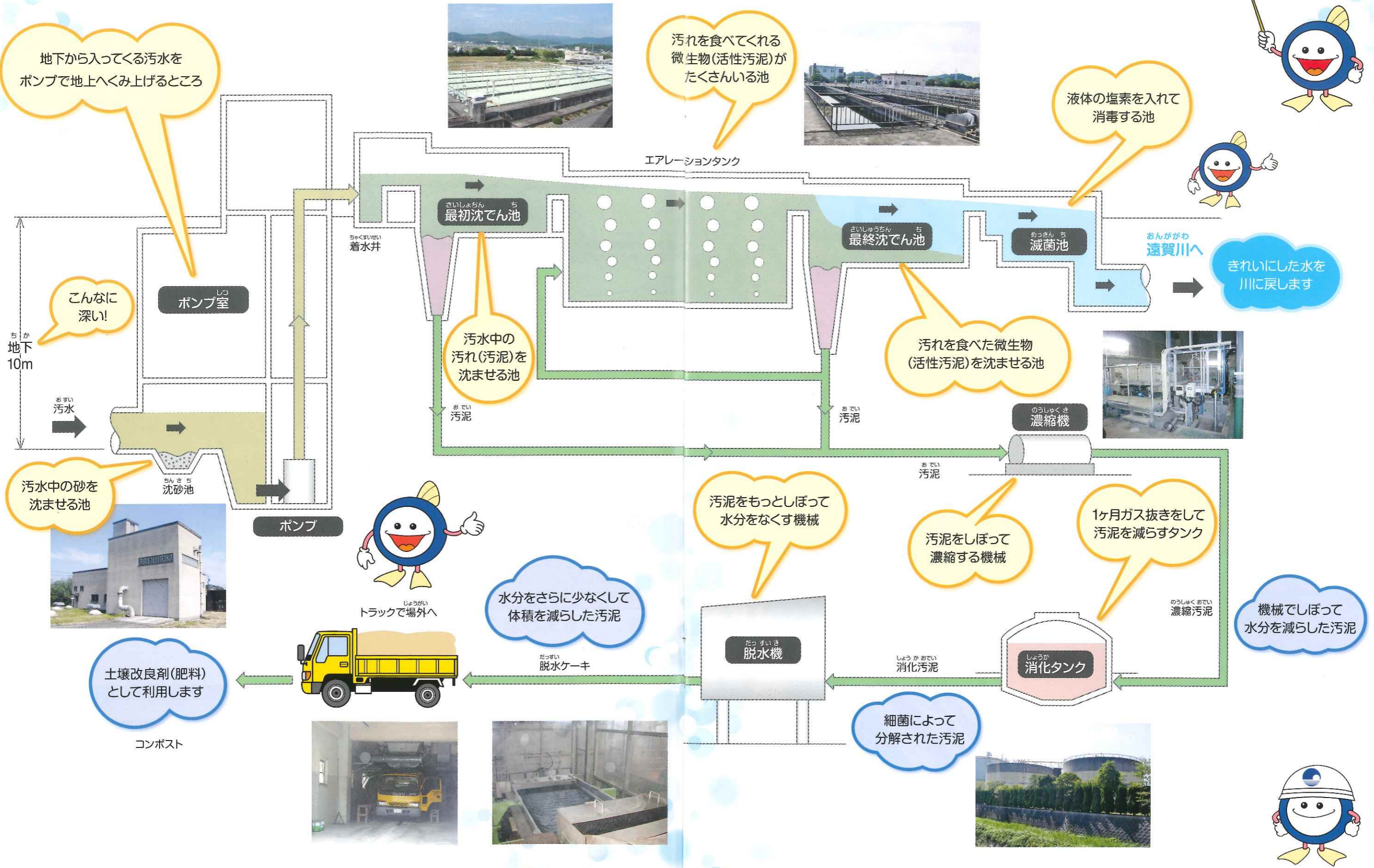
【飯塚終末処理場フロー図】
