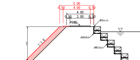
仮設道路A
