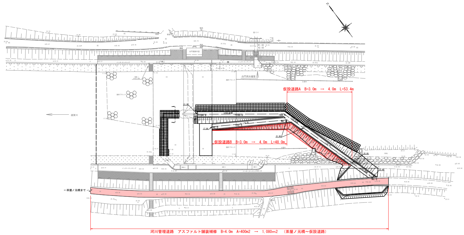
仮設道路B
