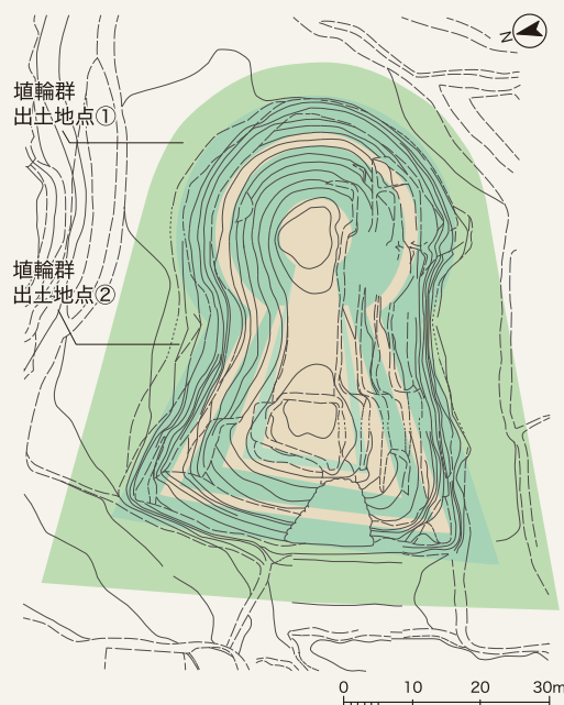
墳丘測量図(1/1200)
